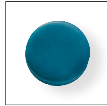
Indicolite
